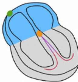
Potentiel électrique en divers endroits du cœur et électrocardiogramme (ECG)
