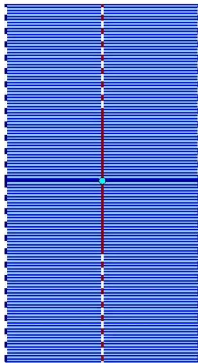
Un polydisque dans un espace vectoriel normé de rang supérieur
