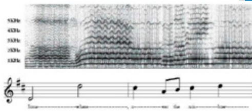
Représentations temps-fréquence de signaux sonores
