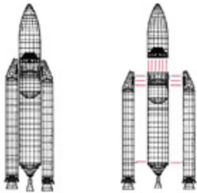
Décomposition de domaine: géométries
