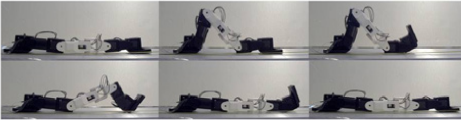
FIGURE 7 – Décomposition du cycle du mode chenille sur le robot.
