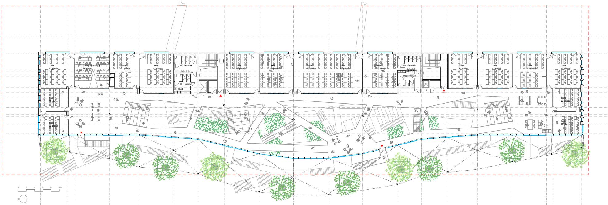
Ci-dessus : Plan d'un étage courant (R+3) ©SFA-OXO-NLA-DR Ci-dessous : Plan du rez-de-chaussé (RDC) ©SFA-OXO-NLA-DR
